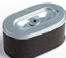
Vzduchový filtr EX27 dual objednací číslo: 279-32607-17 rozměry (DxŠxV): 145 x 85 x 70 mm
